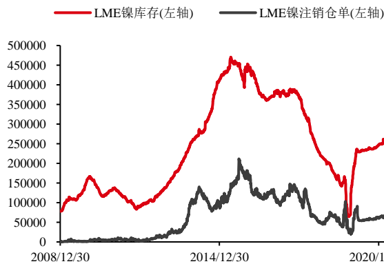
图 5:LME 镍库存 | 单位: 吨
